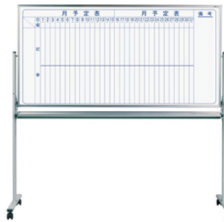
MV36TDMN G ¥63,000 外形寸法 / W1926×D610×H1840 板面寸法 / W1810×H910 有効寸法 / W1770×H870
